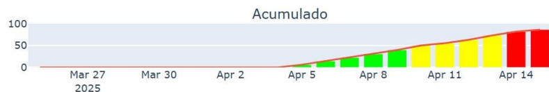
Modelo predictivo de Goidanich (Datos: estación SIAR Borja)
